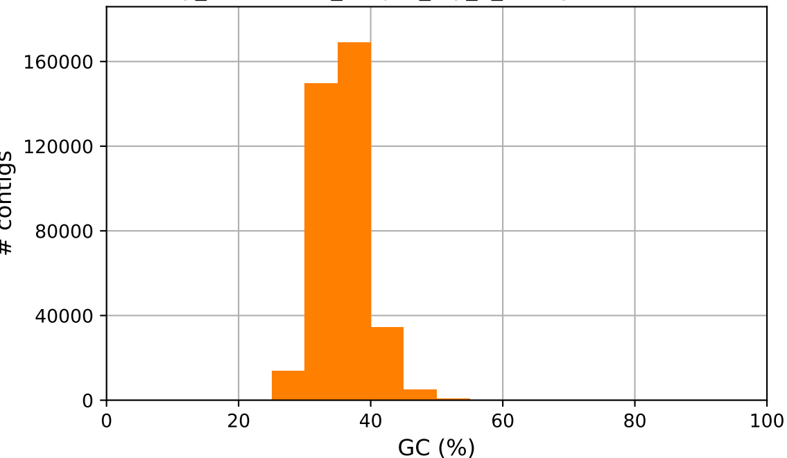
Oly_Redundans_Output_Try_2_contigs GC content
