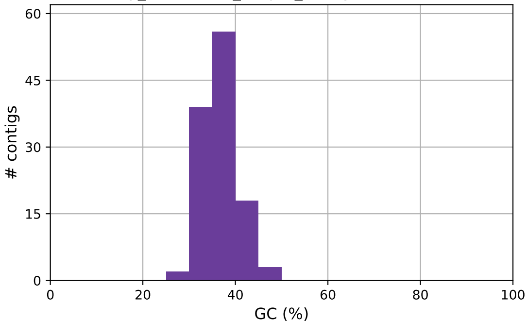
Oly_Redundans_Output_contigs GC content
