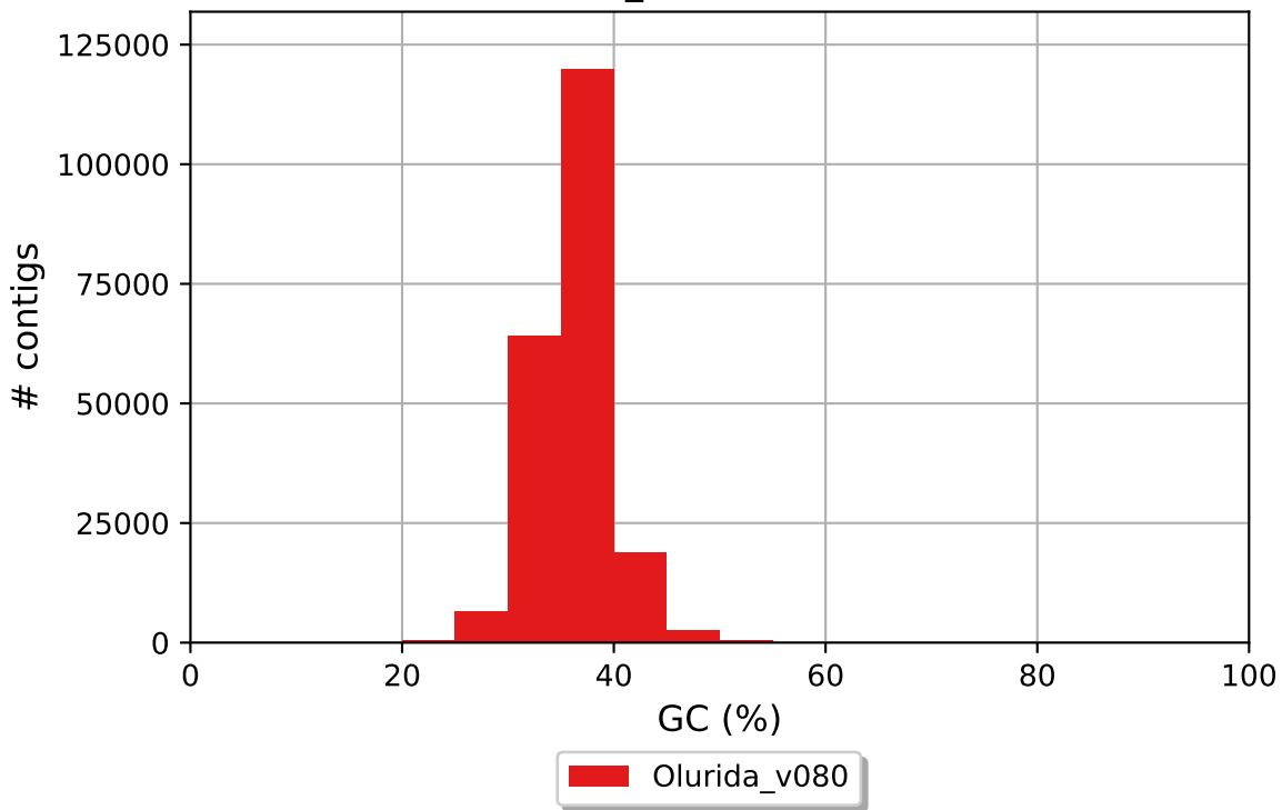
Olurida_v080 GC content
