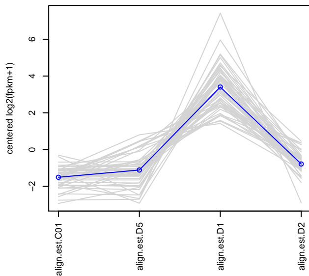
subcluster_2_log2_medianCentered_fpkm.matrix, 48 trar
