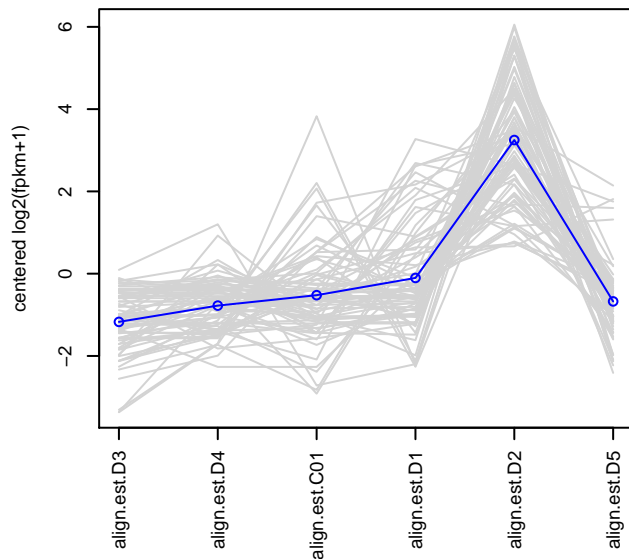
subcluster_7_log2_medianCentered_fpkm.matrix, 76 trar
