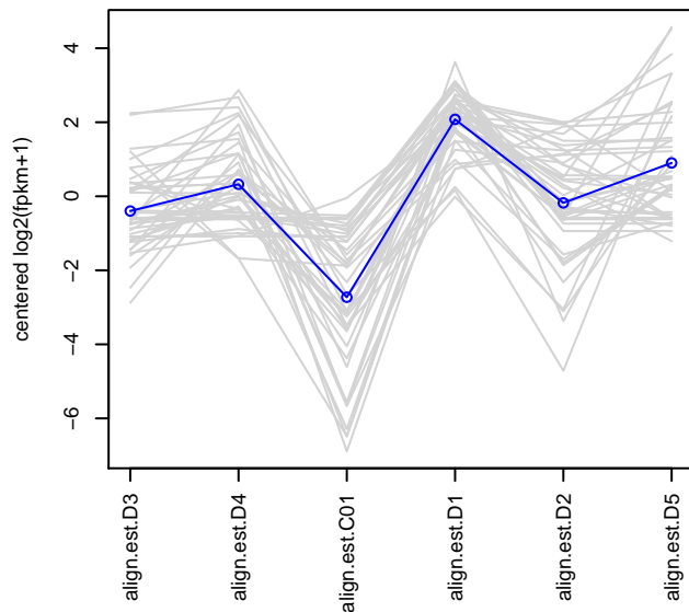
subcluster_9_log2_medianCentered_fpkm.matrix, 43 trar
