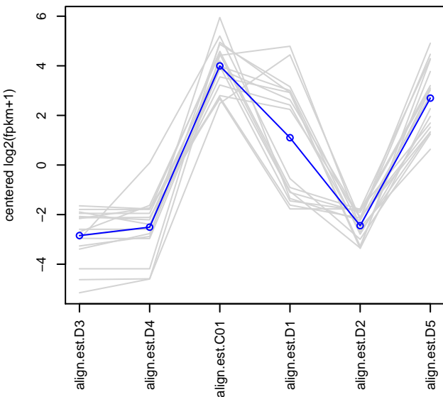
subcluster_8_log2_medianCentered_fpkm.matrix, 17 trar
