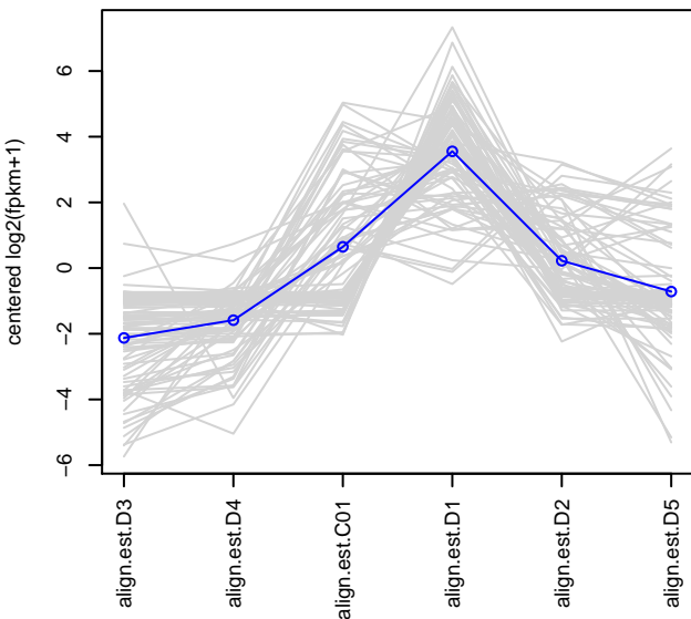
subcluster_6_log2_medianCentered_fpkm.matrix, 86 trar
