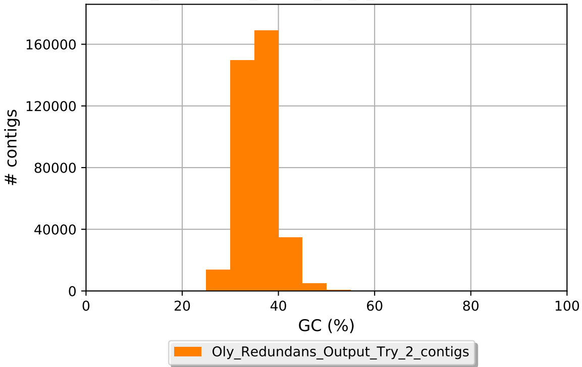
Oly_Redundans_Output_Try_2_contigs GC content
