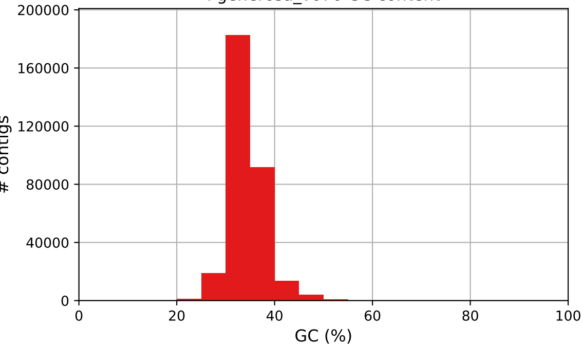
Pgenerosa_v070 GC content
